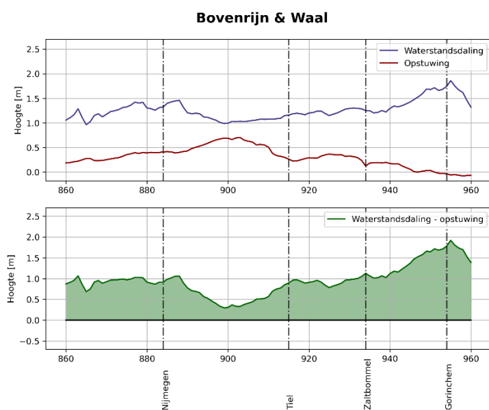
Figuur 2 - Waterstandsdingaling door rivierverruiming en opstuwung door vegetatie gecombineerd voor de Bovenrijn en Waal.
